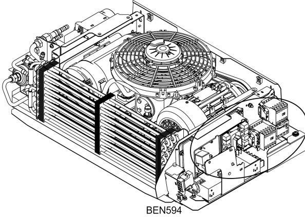
Ilustración 11. Ubicación de los fusibles (cubierta del condensador retirada)
