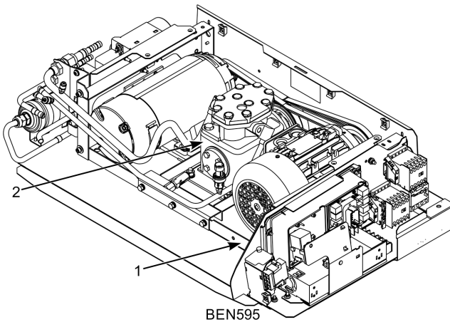
Ilustración 12. Ubicaciones de los números de serie del condensador y del compresor eléctrico
